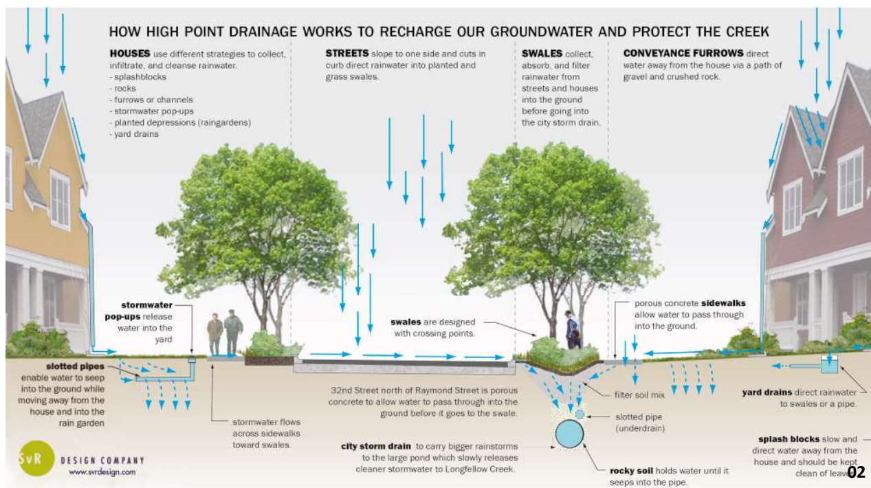
01_Comportament drenatge previ i posterior a l'urbanització 02_Treball dels SUDS evitant l'acumulació d'aigua en superfície
